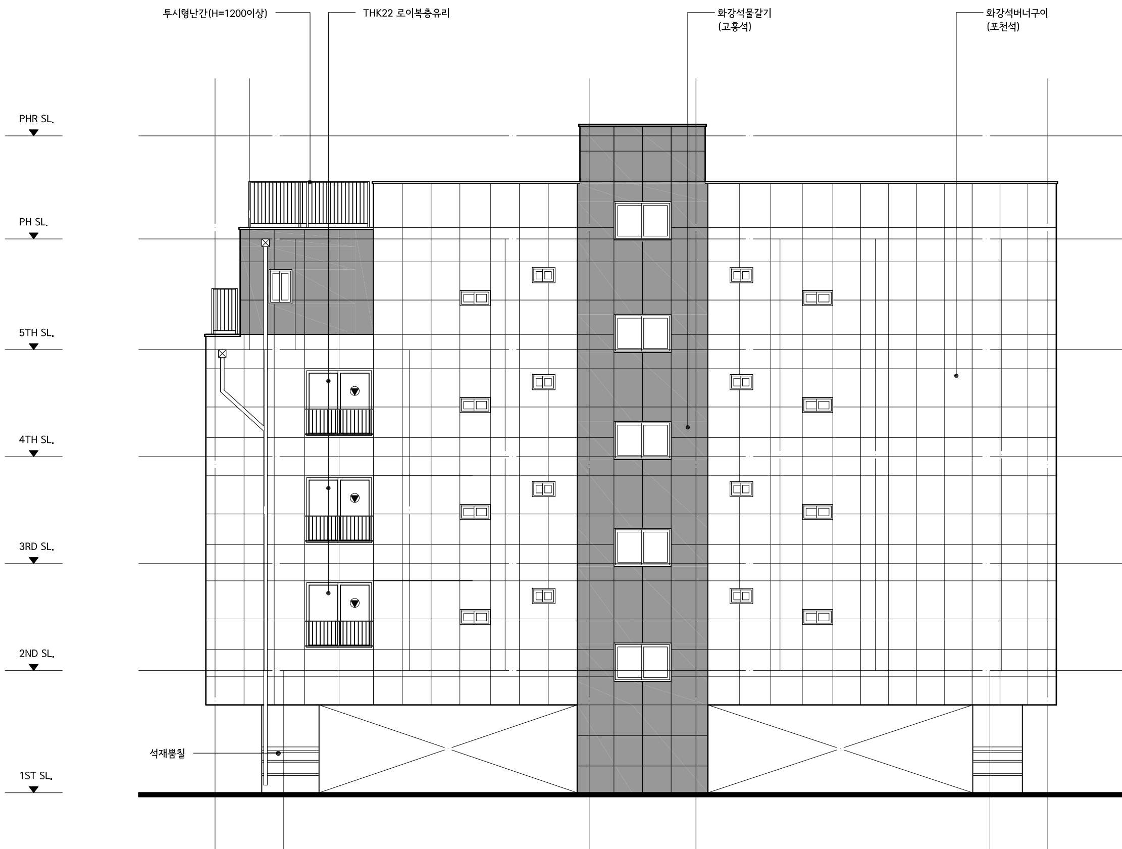
서 측 면 도 SCALE = 1/100
